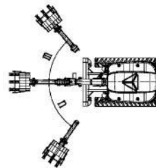
Diagramm der Hauptabmessungen
